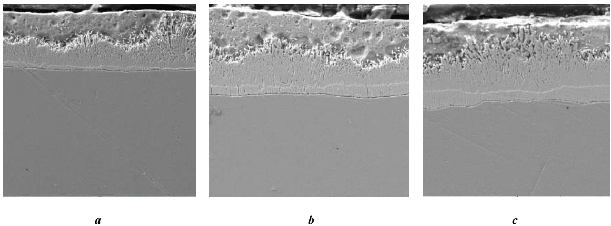
Рис. 5. Микроструктура покрытия на стали C235 (Si=0,02 %), ×1000, время выдержки: a – 1 мин; b – 3 мин; c – 5 мин Fig. 5. The microstructure of a coating on S235 steel (Si=0.02 %), ×1000, holding time: a – 1 min.; b – 3 min.; c – 5 min.
