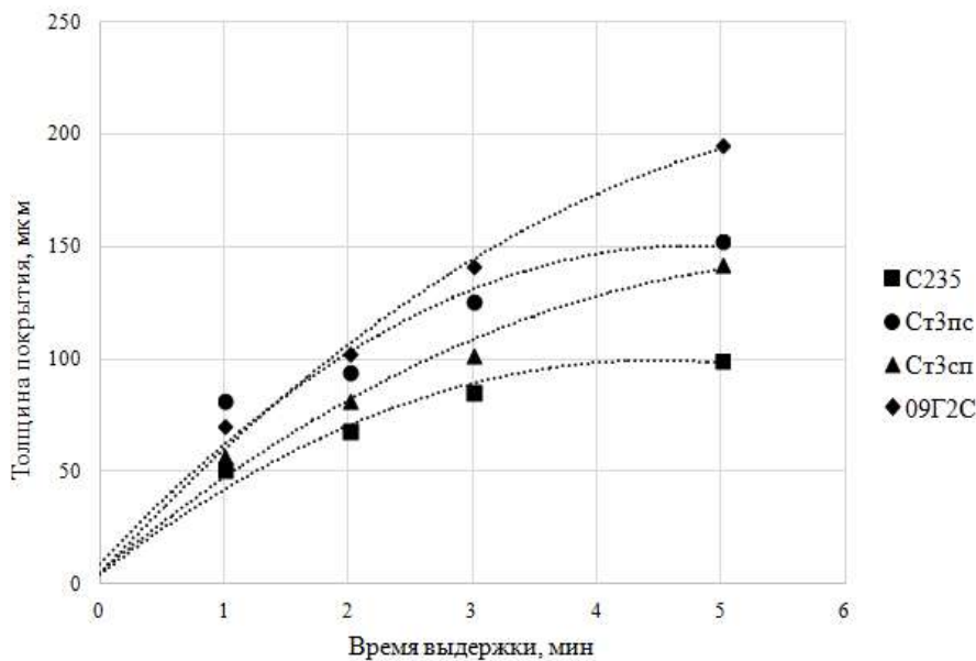
Рис. 3. Зависимость толщины покрытия от времени выдержки образцов в расплаве для сталей С235, Ст3пс, Ст3сп и 09Г2С
