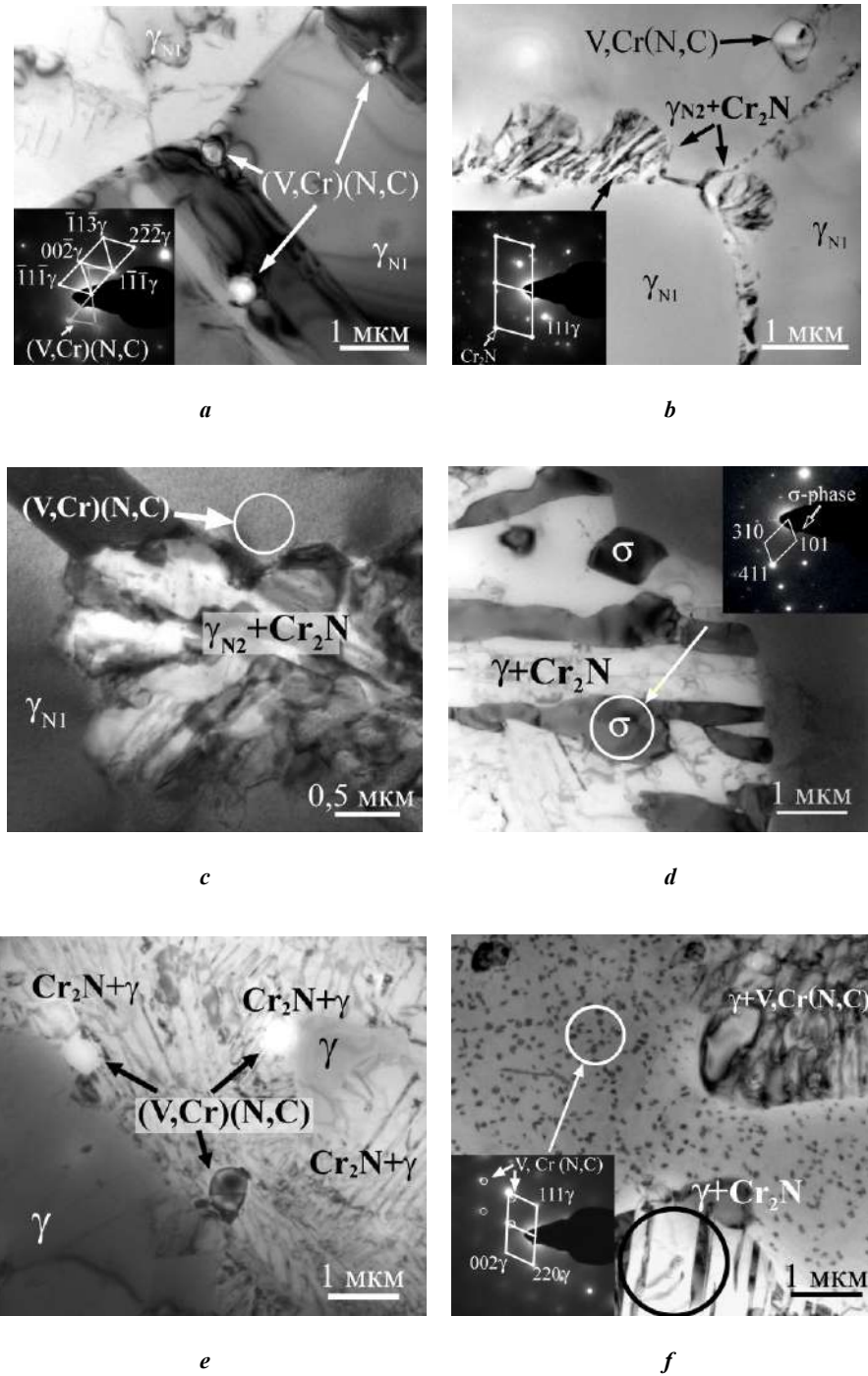
Рис. 3. Светлопольные ПЭМ-изображения микроструктуры стали Fe-19Cr-22Mn-1,5V-0,3C-0,86N после закалки (а) и после старения (б–ф) по режимам:
