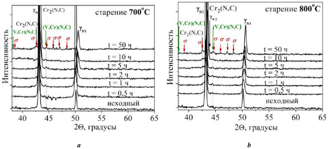
Рис. 1. Влияние продолжительности старения при температурах 700 °С (а) и 800 °С (b) на вид рентгенограмм для стали Fe-19Cr-22Mn-1,5V-0,3C-0,86N Fig. 1. The influence of duration of aging at the temperature of 700 °С (a) and 800 °С (b) on the form of X-ray patterns for Fe-19Cr-22Mn-1.5V-0.3C-0.86N steel
