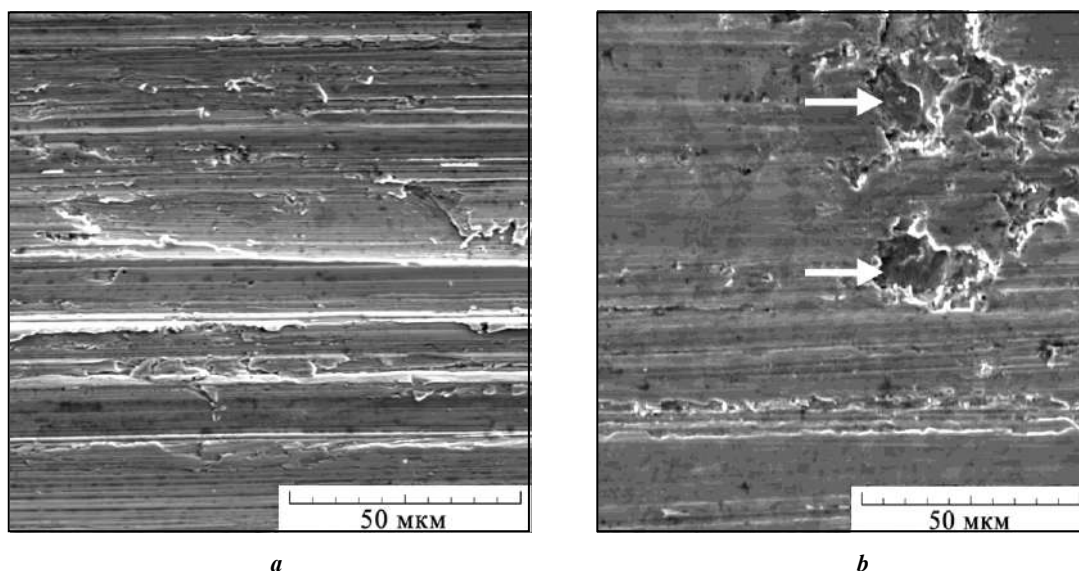
Рис. 4. Поверхности абразивного изнашивания (РЭМ) после испытаний по корунду покрытий: а – ПГ-СР2; б – ПГ-СР2+Cr 3 C 2
