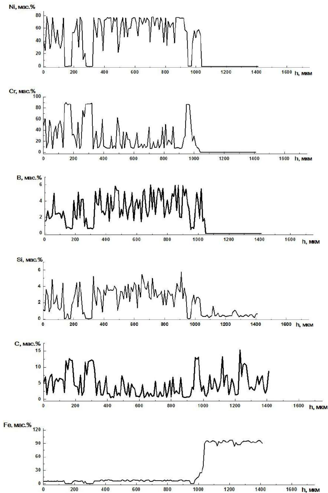
Рис. 2. Распределение химических элементов по глубине наплавленного лазером покрытия NiCrBSi–Cr 3 C 2 Fig. 2. Chemical elements depth distribution in the NiCrBSi–Cr 3 C 2 laser-cladded coating
