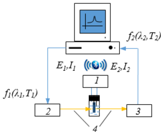
Рис. 3. Схематическое изображение измерительной системы для спектроскопического анализа: 1 – потенциостат; 2 – источник света; 3 – спектрометр; 4 – оптоволокно
