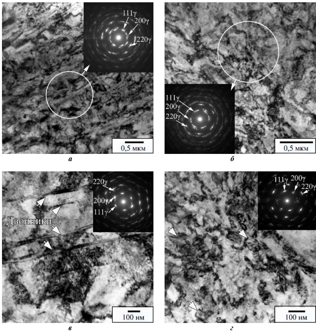
Рис. 2. Микроструктура образцов стали типа 316L после термомеханических обработок по Режиму 1 (а, в) и Режиму 2 (б, г). Светлопольные ПЭМ изображения (а-г) и соответствующие им микродифракционные картины (МД) (вставки на а-г). Стрелки на (г) указывают на рекристаллизованные зерна. МД получены с участков фольг площадью 1,5 мкм 2 (а, б), 1,2 мкм 2 (в) и 0,3 мкм 2 (г)
