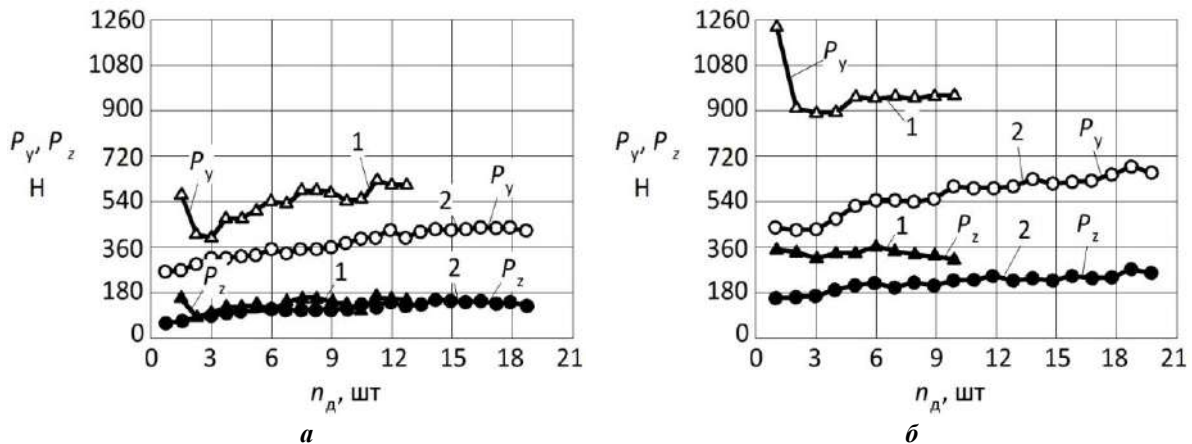
Рис. 2. Зависимости сил резания при шлифовании в течение периода стойкости круга: а – правка новым ПИ; б – правка изношенным ПИ. n_d – количество прошлифованных образцов; 1 – силы после ОП; 2 – силы после УЗП
