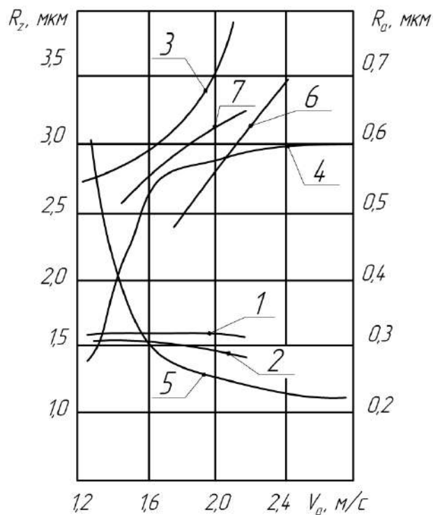
Рис. 1. Шероховатость обработанной поверхности при УЗС в зависимости от изменения V_H , P и материала инструмента (Сплав ВТ3-1): 1 – P=0,2/0,1 МПа; брусок 63СМ20СТ17К8; 2 – P=0,3/0,15 МПа; брусок 63СМ20СТ17К8; 3 – P=0,3/0,13 МПа; брусок 63С4ПСМ17К8; 4 – P=0,2/0,1 МПа; брусок 63СМ10СТ17К8; 5 – P=0,3/0,15 МПа; брусок 63СМ10СТ17К8; 6 – P=0,2/0,1 МПа; брусок 63С5ПСТ17К8; 7 – P=0,3/0,15 МПа; брусок 63С5ПСТ17К8
