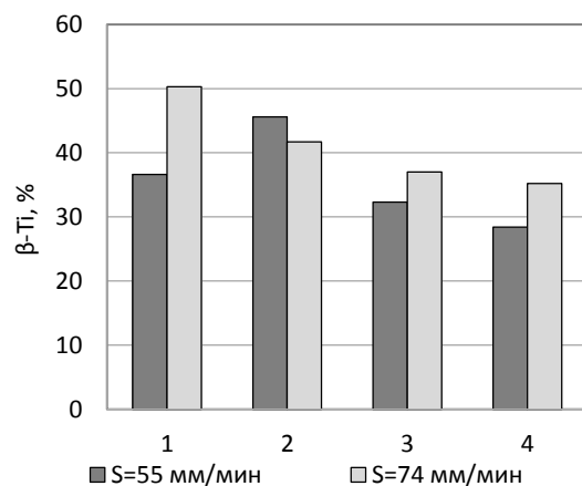
Рис. 6. Диаграмма изменений соотношения фаз при обработке заготовок из ВТ6 на режимах:
