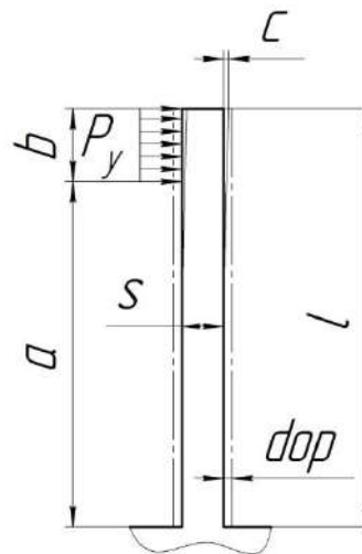
Рис. 2. Схема нагружения, при котором набор параметров принимается в работу
