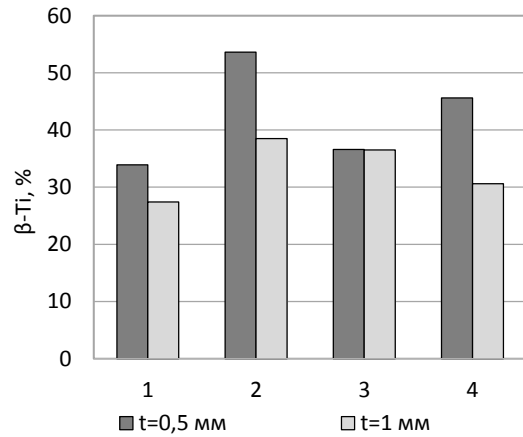
Рис. 5. Диаграмма изменений соотношения фаз при обработке заготовок из ВТ6 на режимах:
